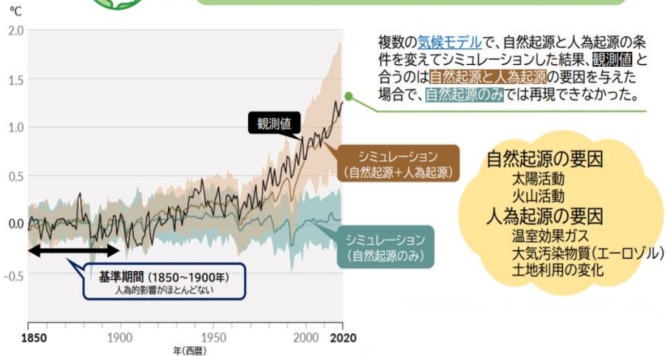
図 1850～1900年を基準とした世界平均気温の変化 陰影部は可能性が非常に高い範囲。出典:AR6 WG1 図 SPM.1(b)
