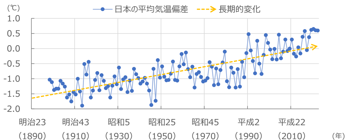
図 24 日本の年平均気温偏差の推移
