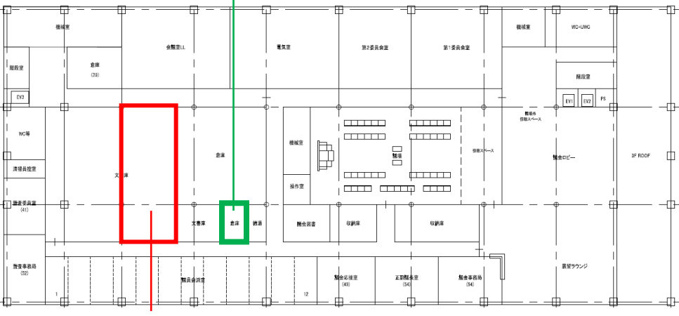
4階平面図
