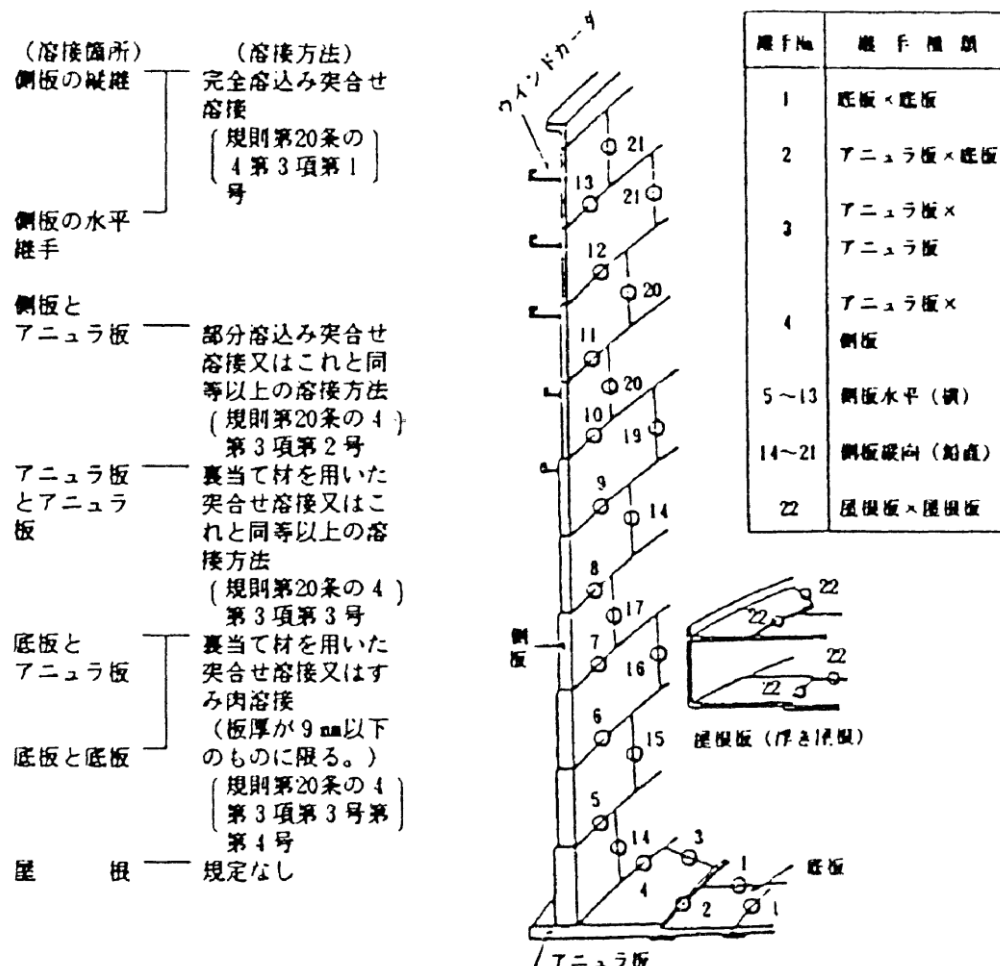
第3-5-1図 浮屋根式タンクの溶接継手
