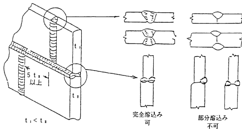
第3-5-2図 側板の溶接
