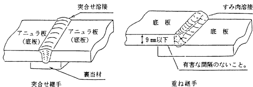
第3-5-4図 アニュラ板、底板の溶接
