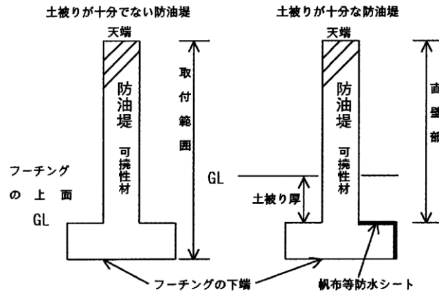
第3-2-1図 可撓性材の取り付け範囲
