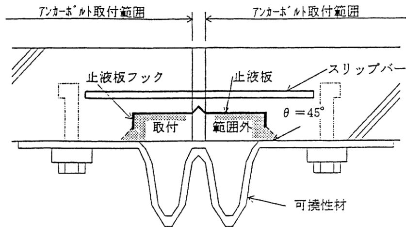
第3-2-2図 アンカーボルト取り付け範囲 (防油堤目地部を上から見た図)
