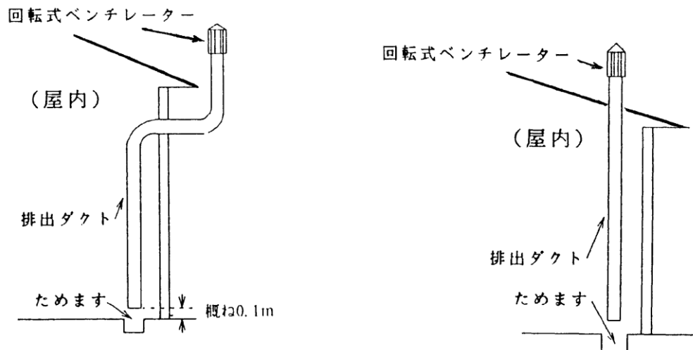
第17-6図 強制排出設備の例
