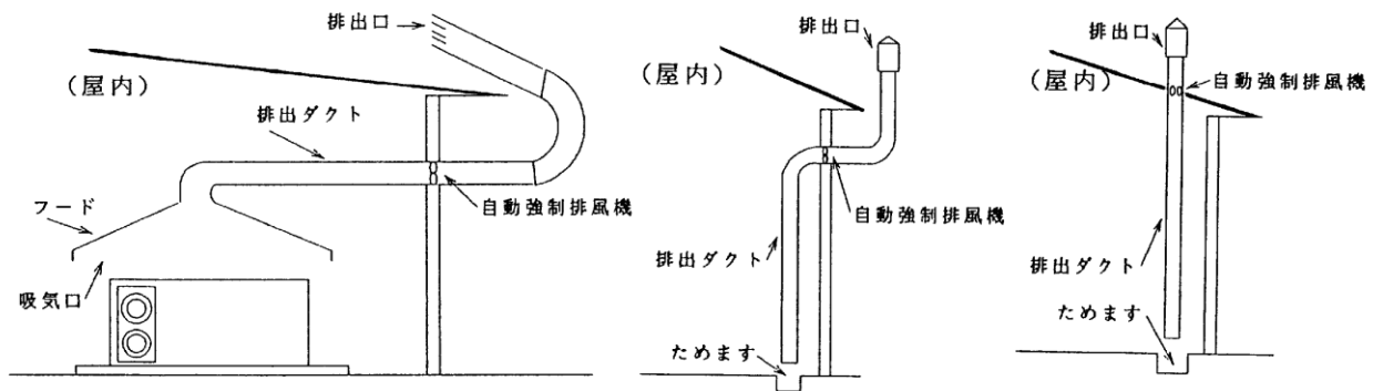
第17-5図 自動強制排出設備の例
