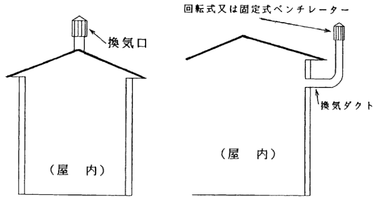
第17-2図 強制換気設備の例
