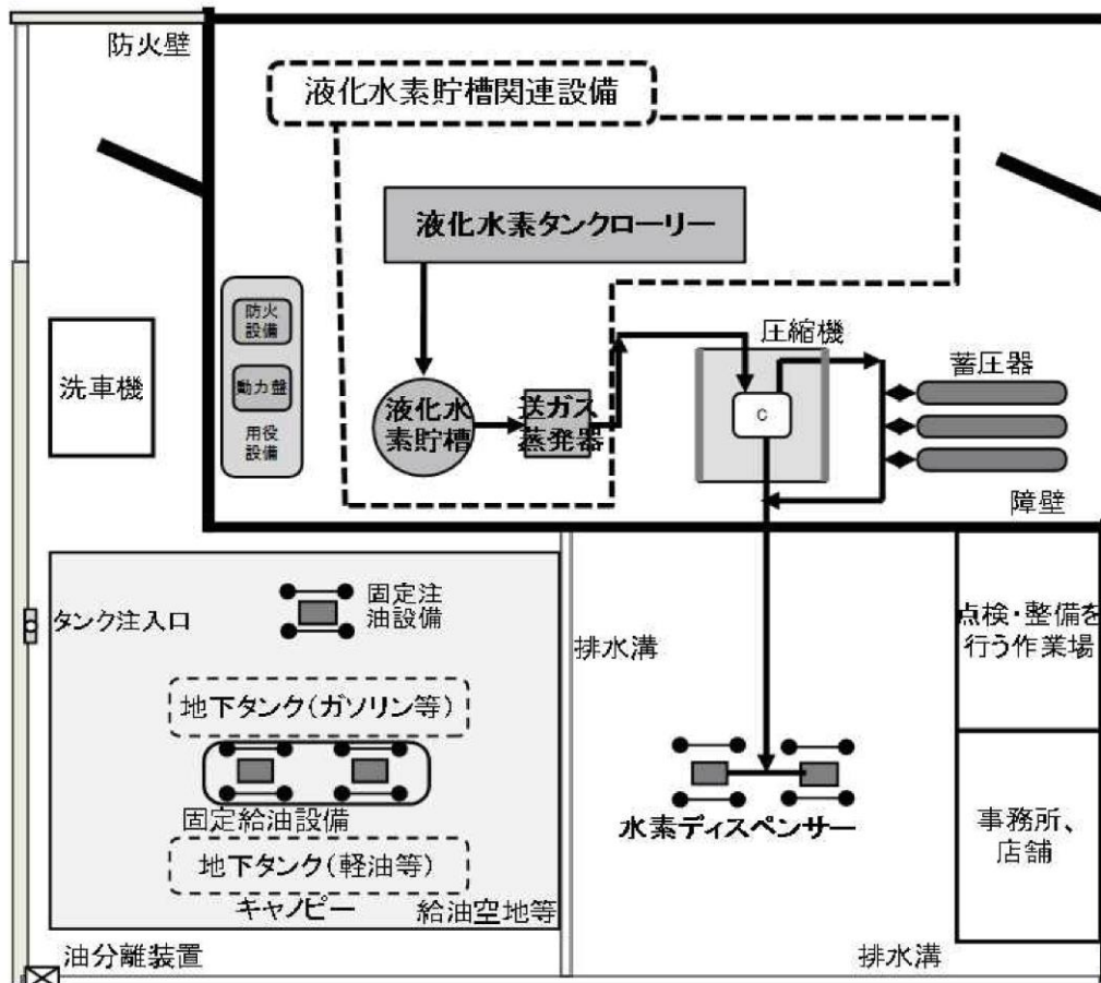
第13-64図 液化水素の貯槽を設置する圧縮水素充填設備設置給油取扱所の設置例
