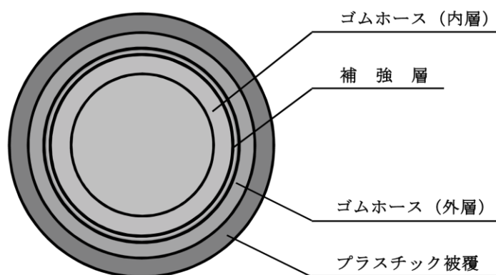
第13-11図 プラスチックで被覆された給油ホースの構造 (断面)
