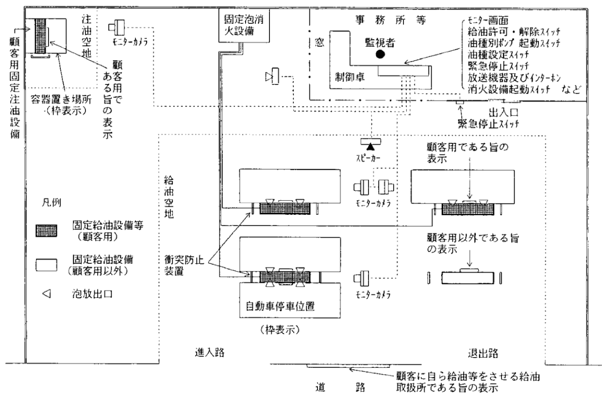
第13-82図 セルフ給油取扱所の設置例
