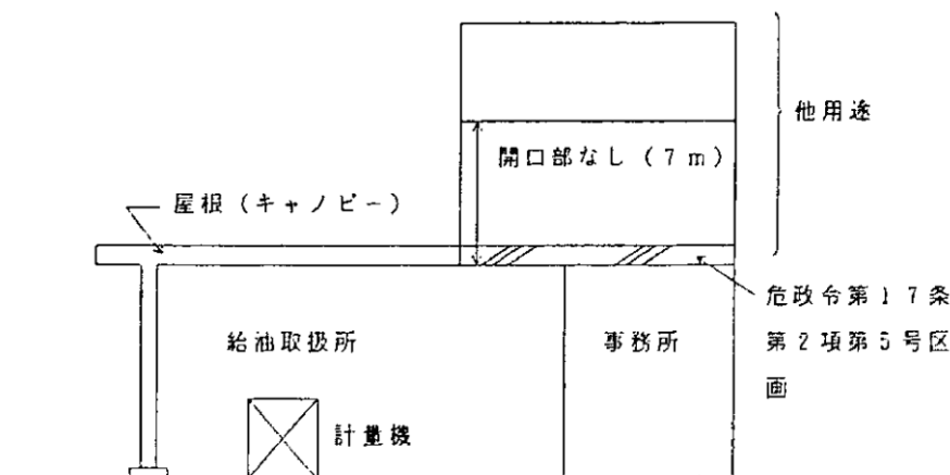
第13-37図 給油取扱所の屋根部分を不燃材料とすることができる例
