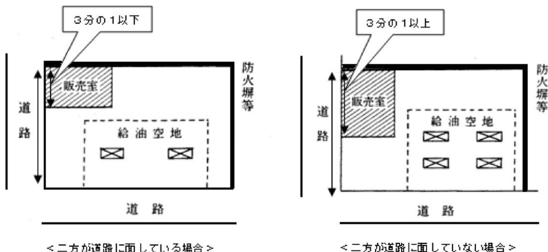
第13-33図 二方開放の例
