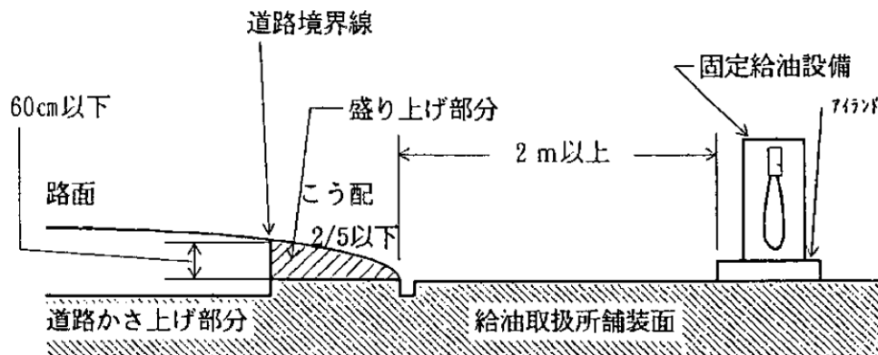
第13-7図 周囲の地盤面との関係
