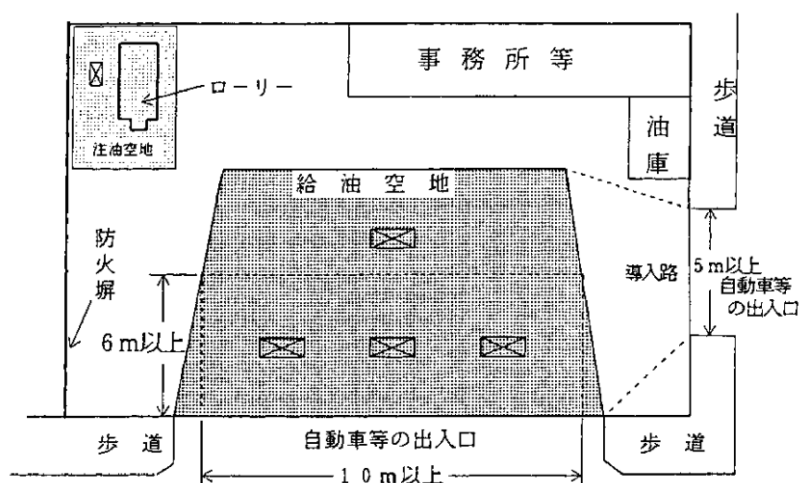
第13-2図 給油空地の例
