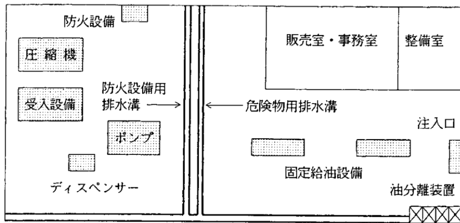
第13-57図 危険物用と防火設備用の排水溝を別々に設置した例
