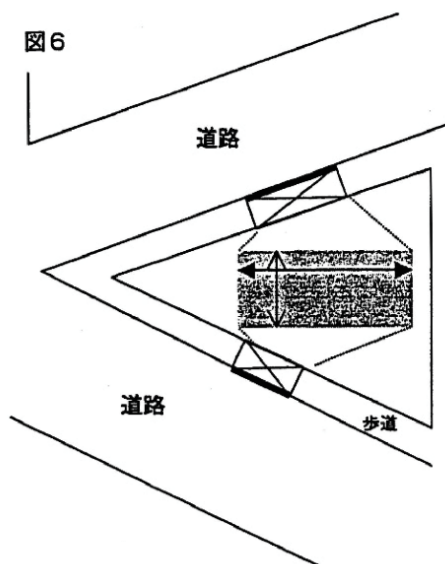
第13-5図 給油空地の例示
