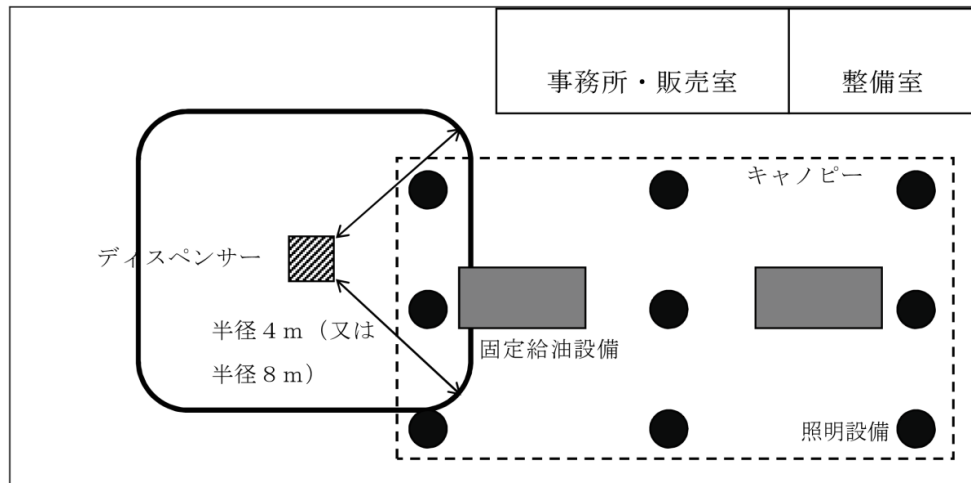
第13-46図 電気設備に防爆措置が必要な範囲(デイスペンサー外面から)
