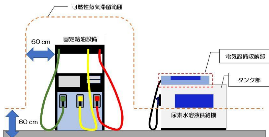
第13-21図 尿素水溶供給機（電動ポンプにより払い出すタイプ）
