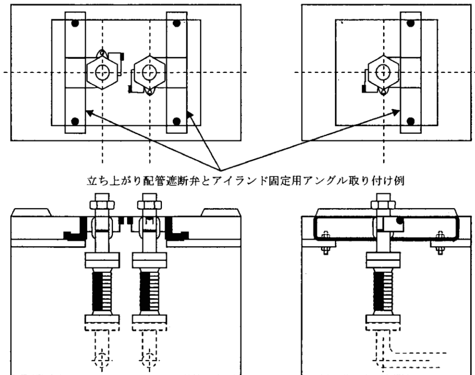
第13-80図 立ち上がり配管遮断弁の取り付け例
