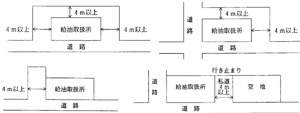
第13-16図 自動車が出入りする側の例
