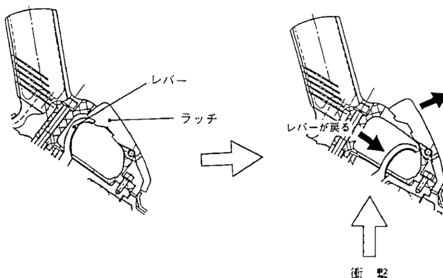
第13-76図 脱落時停止制御装置の作動例
