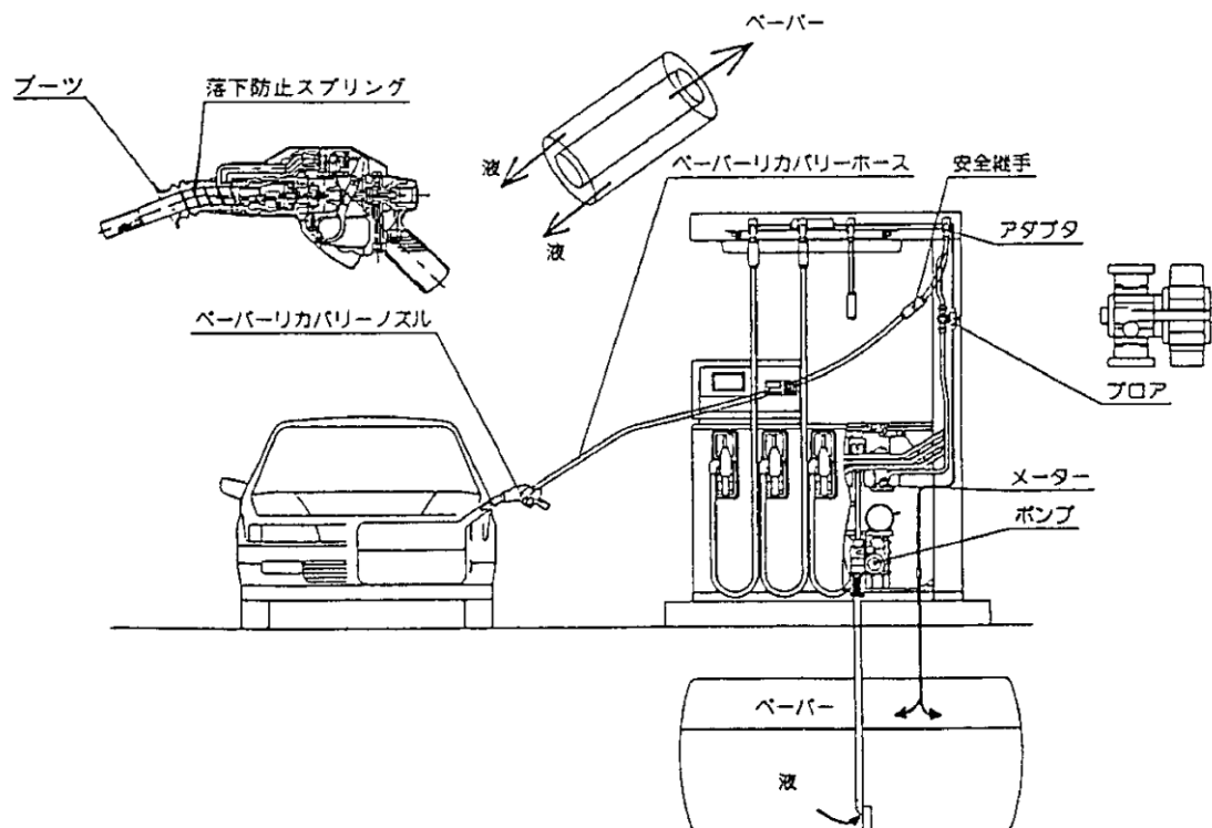
第13-77図 可燃性蒸気回収装置の構造例
