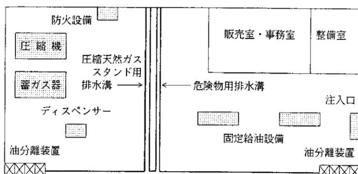
第13-52図 危険物用と圧縮天然ガススタンド用の排水溝を別々に設置した例
