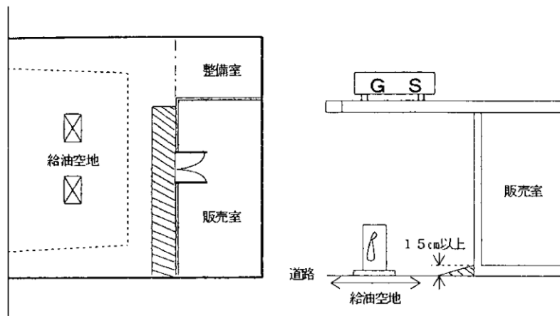
第13-15図 コンクリート製スロープ設置例
