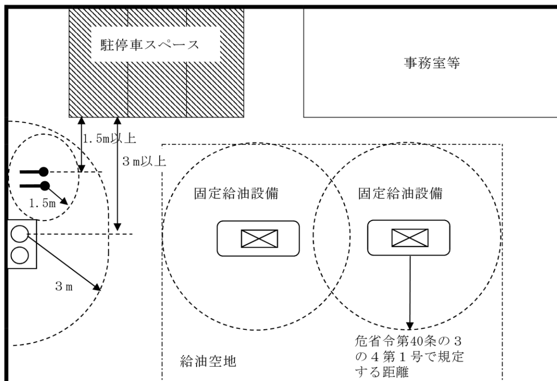
第13-30図 駐停車スペースの例
