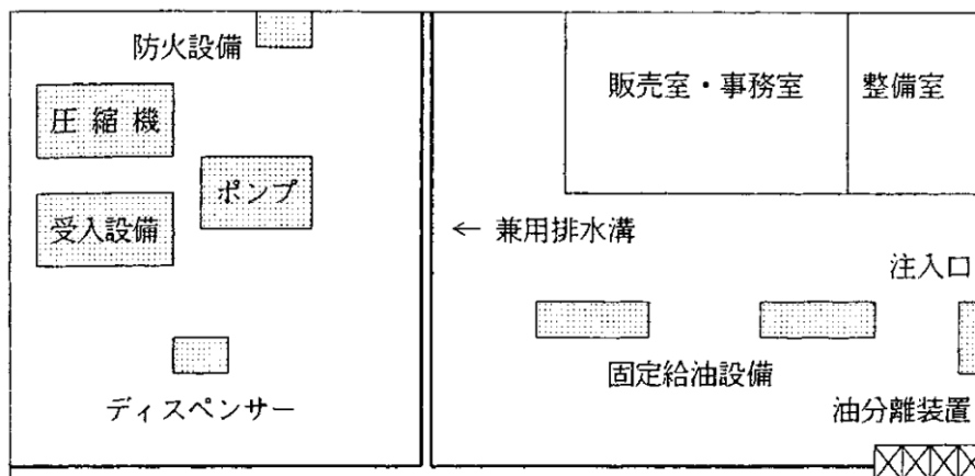
第13-56図 危険物用と防火設備用の兼用排水溝の設置例
