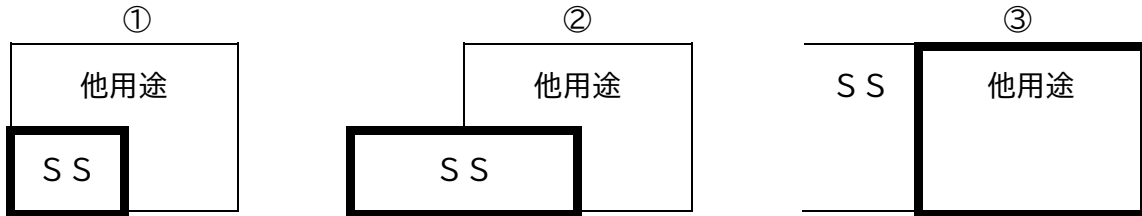
第13-31図 建築物内に設置されている給油取扱所の例
