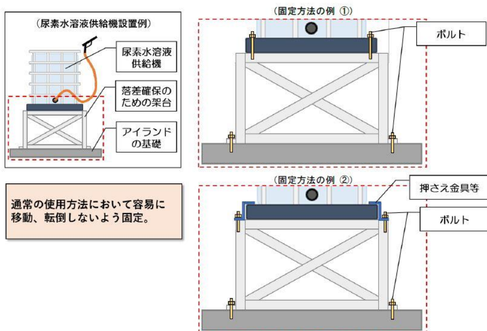
第13-22図 尿素水溶液供給機（重力により払い出すタイプ）
