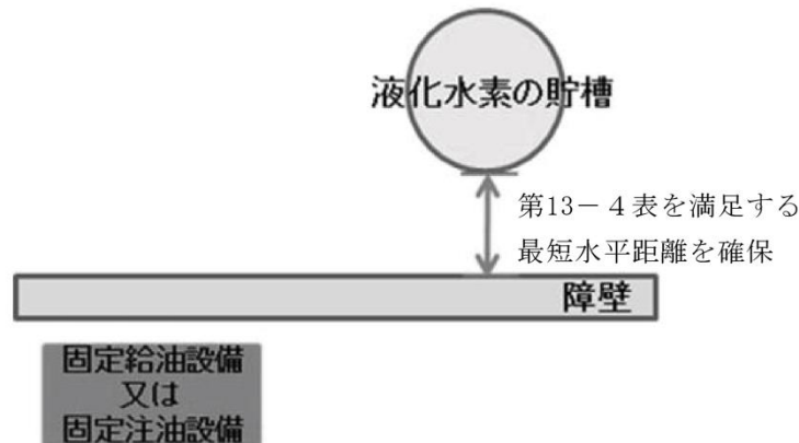
第13-61図 障壁から必要な最短水平距離を確保する方法
