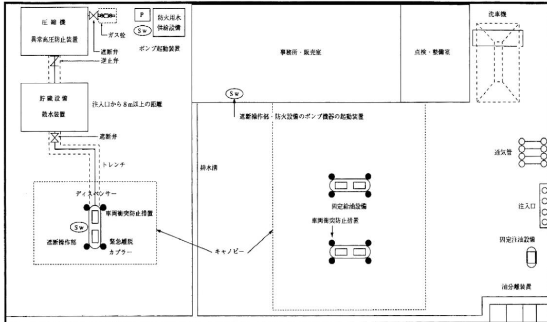
第13-53図 圧縮天然ガス充填設備設置給油取扱所のモデル図
