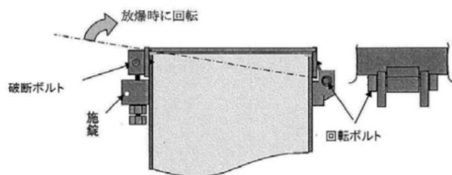
第13-67図 マンホール蓋の固定ボルト
