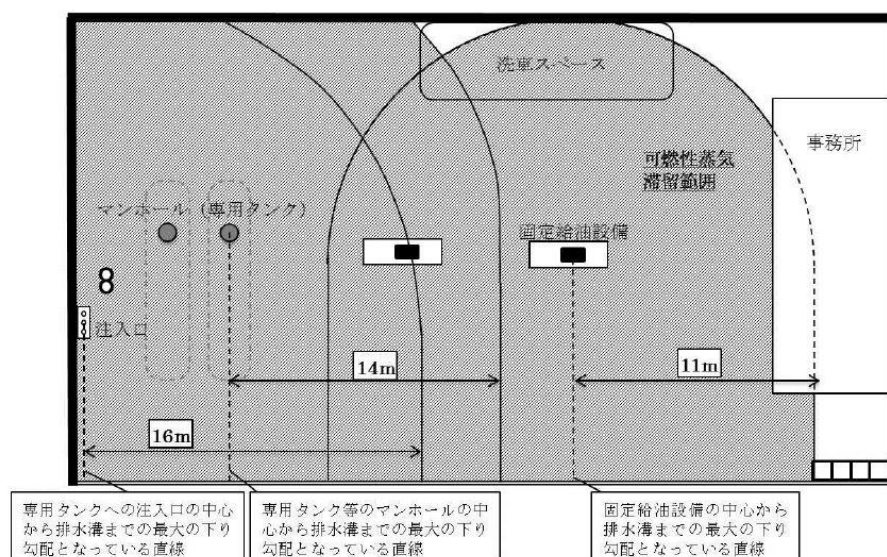
第13-29図 平面図
