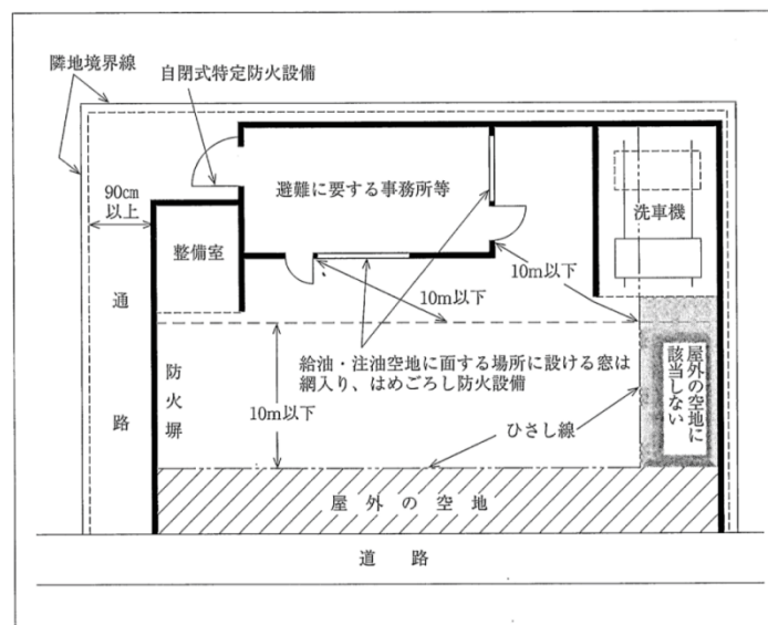
第13-35図 一方開放の屋内給油取扱所
