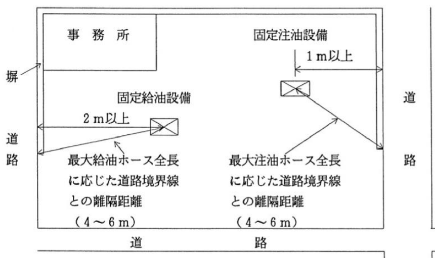
第13-8図 道路境界線に塀又は壁を設けた場合の固定給油設備等の設置例
