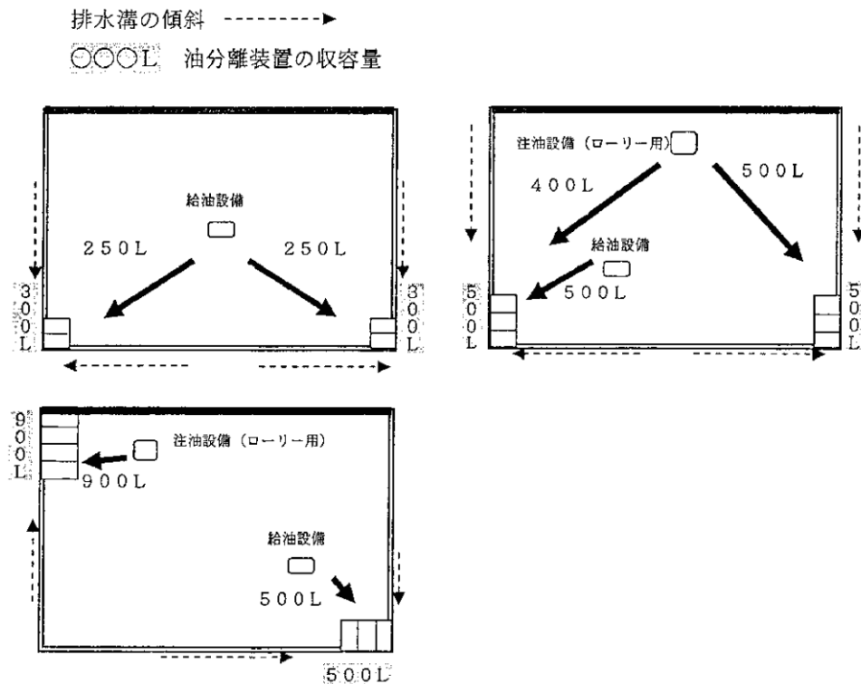
第13－6図 貯留設備の設置例
