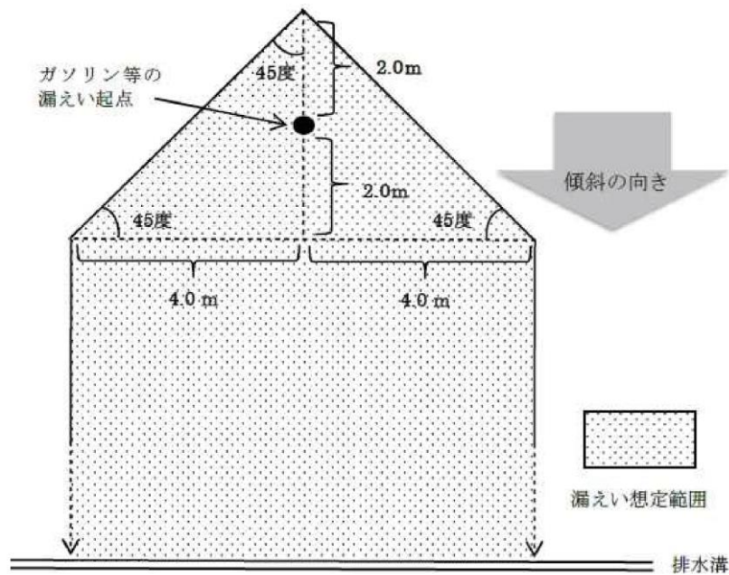
第13-48図 検証に基づく漏えい想定範囲 (条件 給油ノズルの吐出量：毎分50リットル、 傾斜の勾配：1/100～1/75)
