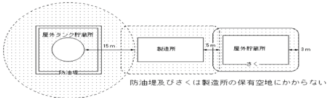
第5－2図 保有空地の例
