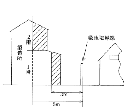
隣地境界線から延焼のおそれのある外壁
