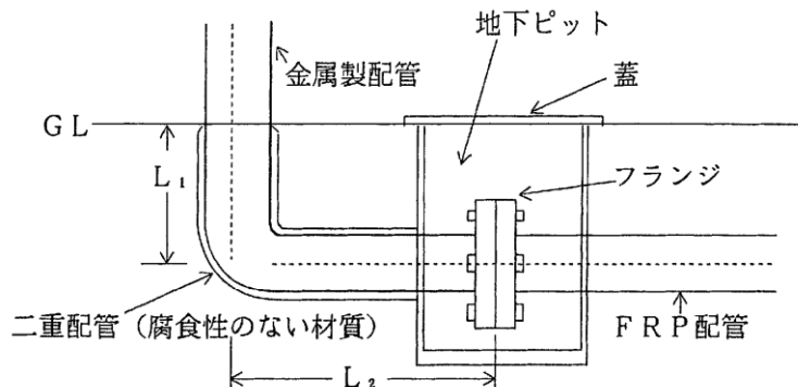
第5-16図 地下ピット内での接続例
