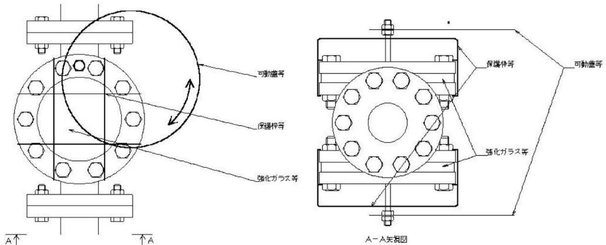
第5-18図 容易に破損しない構造例
