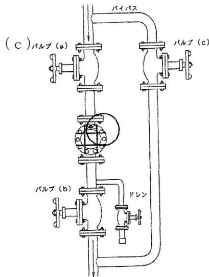
第5-20図 容易に点検整備ができる構造例
