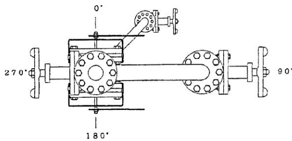
図①： サイトガラスの窓とバルブの方向を変えることにより、安全にバルブ操作が行えるようにした構造例
