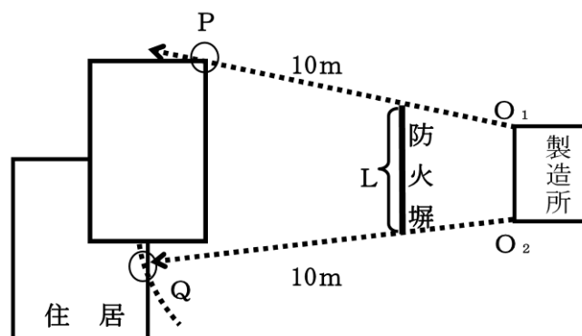
第5-1図 防火上有効な塀
