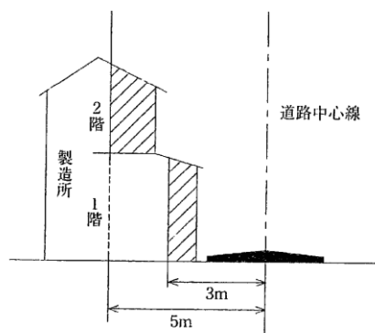
道路中心線から延焼のおそれのある外壁
