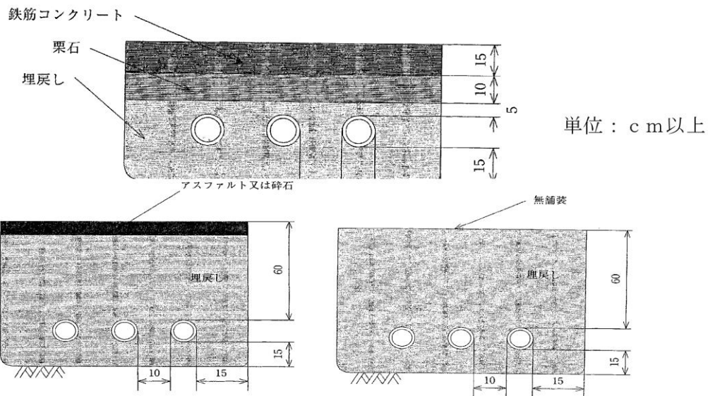
第5-17図 埋設構造例
