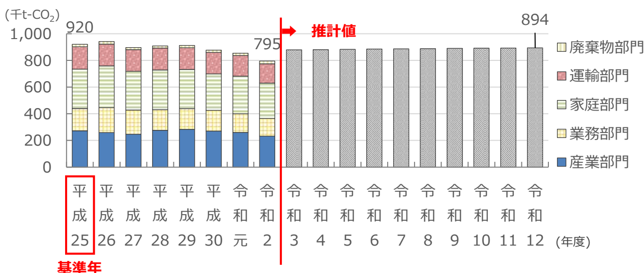
図 29 江別市全体の温室効果ガス排出量の推移
