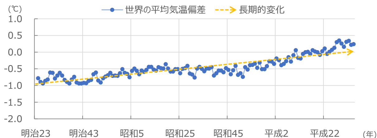
図 23：世界の年平均気温偏差の推移
