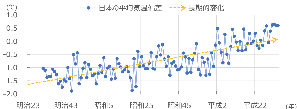
図 24：日本の年平均気温偏差の推移
