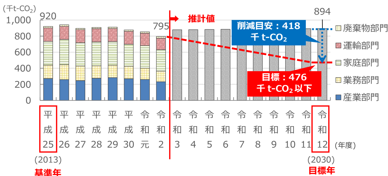
図 37 江別市全体の温室効果ガス排出量の推移
