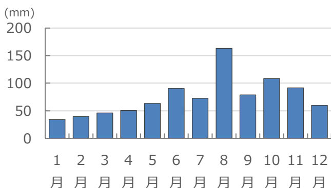
図 10 江別市の平成 29 年～令和 3 年 (2017 年～2021 年) の平均降水量
