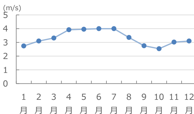
図 12 江別市の平成 29 年～令和 3 年 (2017 年～2021 年) の平均風速
