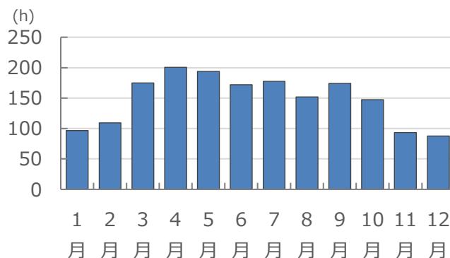
図 9 江別市の平成 29 年～令和 3 年 (2017 年～2021 年) の平均日照時間
