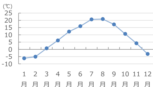
図 8 江別市の平成 29 年～令和 3 年 (2017 年～2021 年) の平均気温
