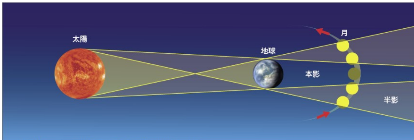
月食の起こる原理 (出典：星空の教科書 (技術評論社))
