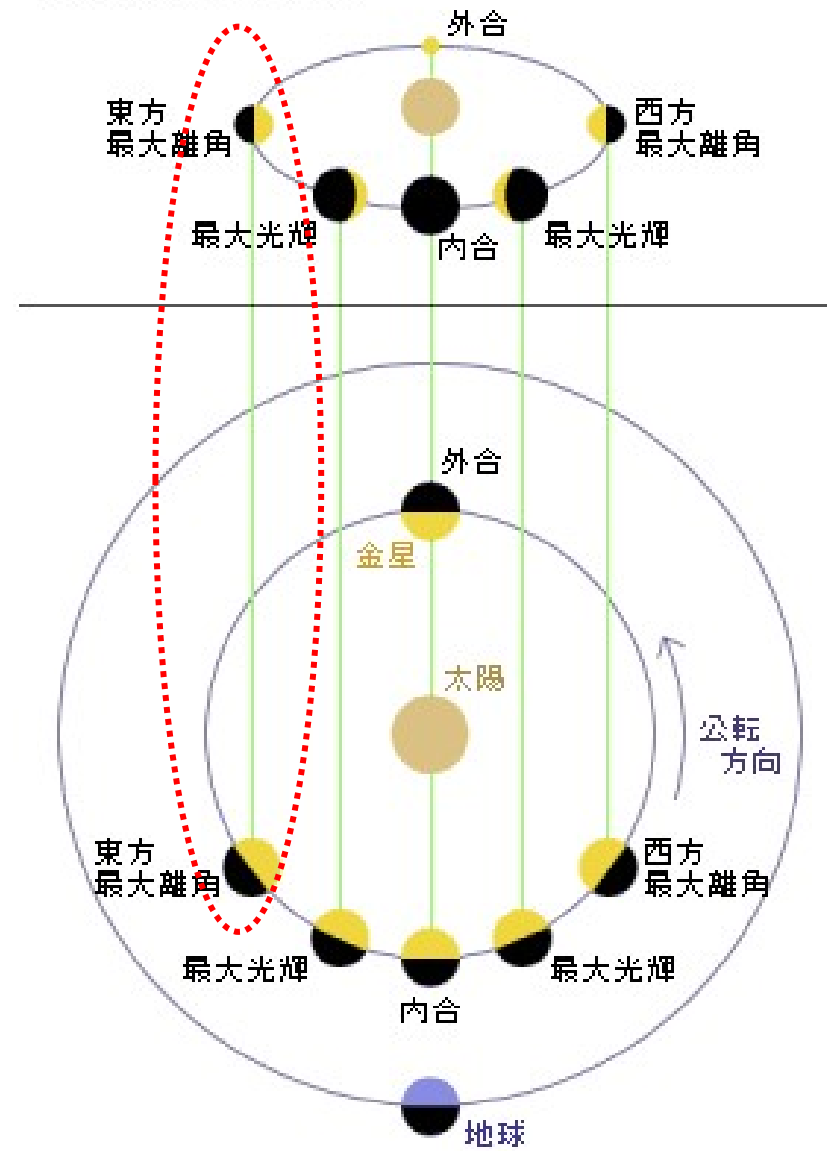
地球・太陽と金星の位置関係
