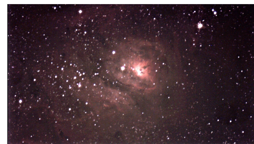
いて座 M8
