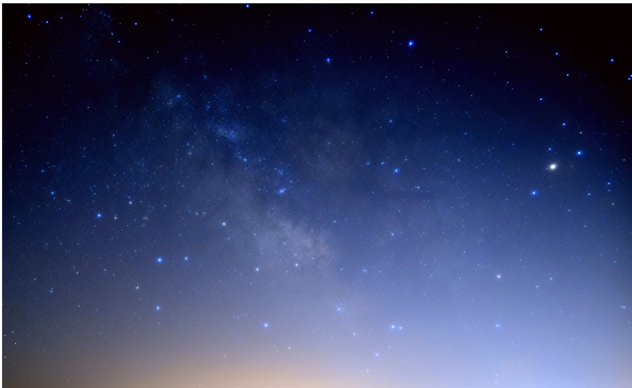
いて座 M17
