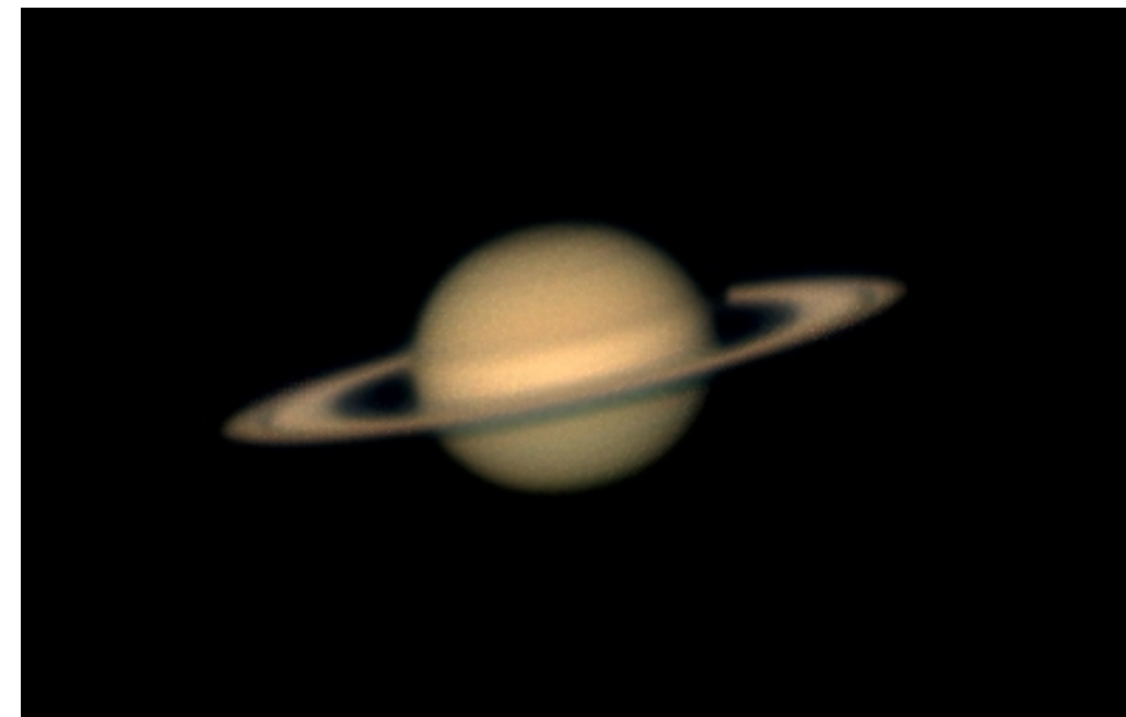
7/9 撮影の土星
