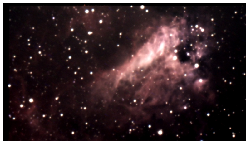
いて座 M17
