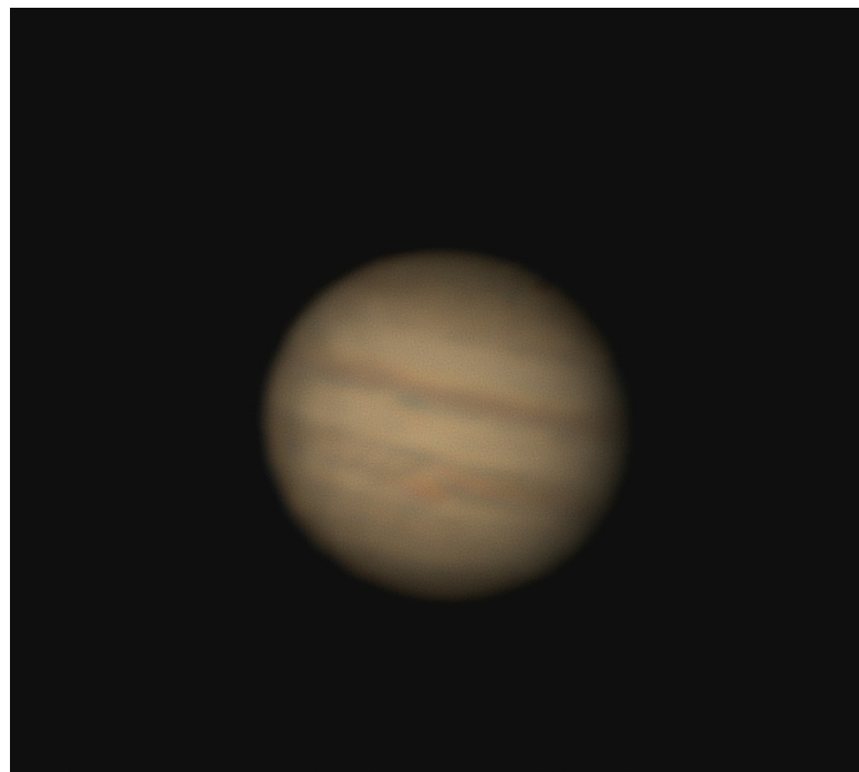
7/9 撮影の木星
