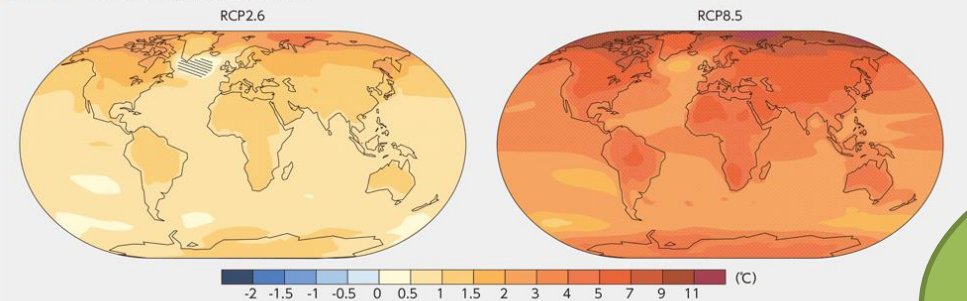
図1-1-3 平均地上気温変化分布 ※ の変化
