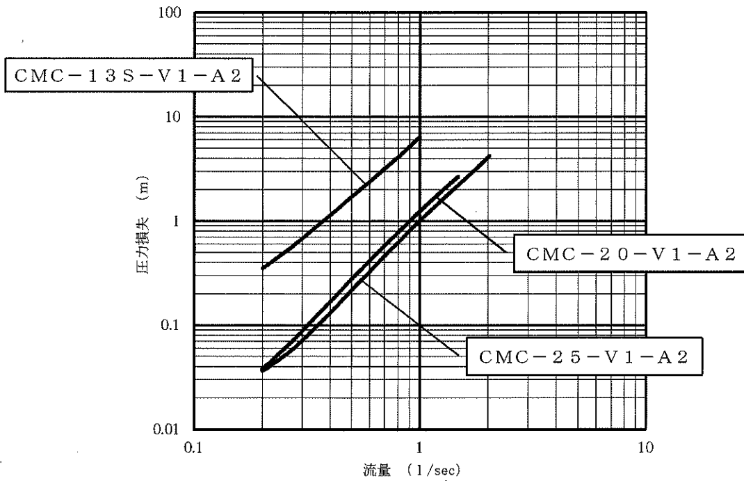
図 損失水頭グラフ
