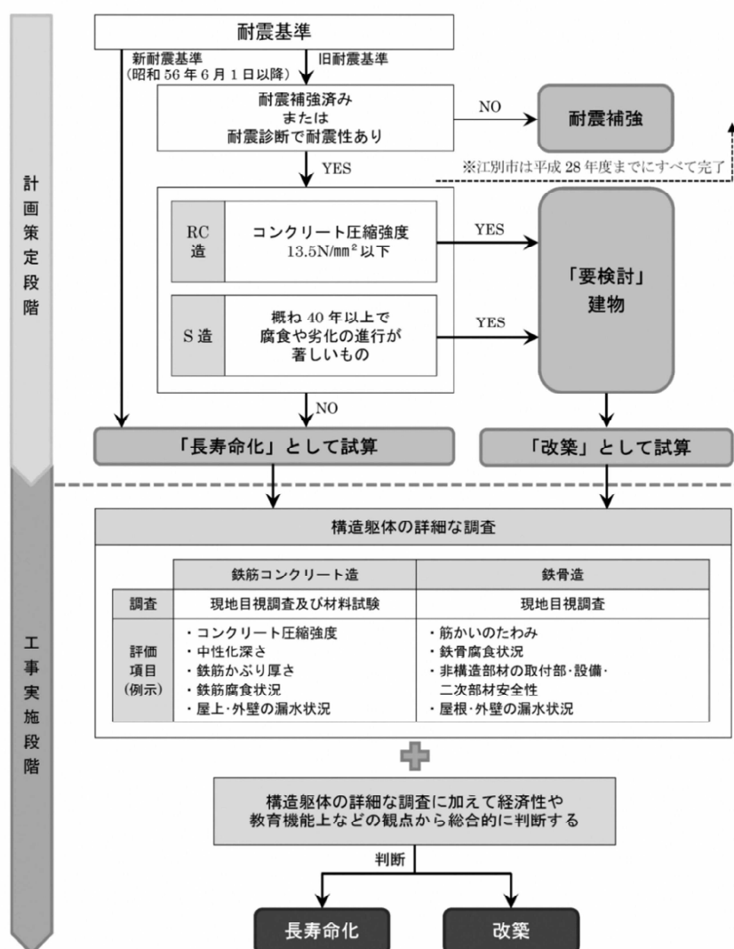
【図表 3-5】長寿命化の判定フロー（「学校施設の長寿命化計画策定に係る解説書」（文部科学省）より）
