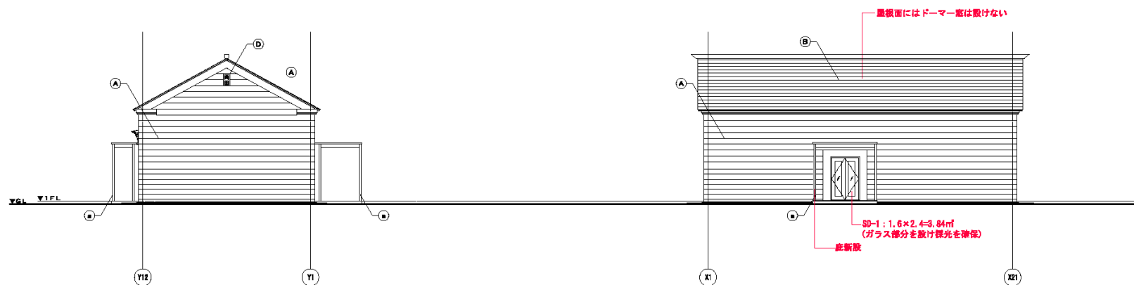
西側立面図 1/100
