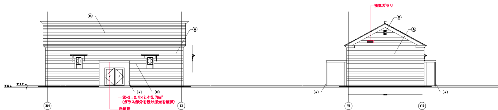
北側立面図 1/100
