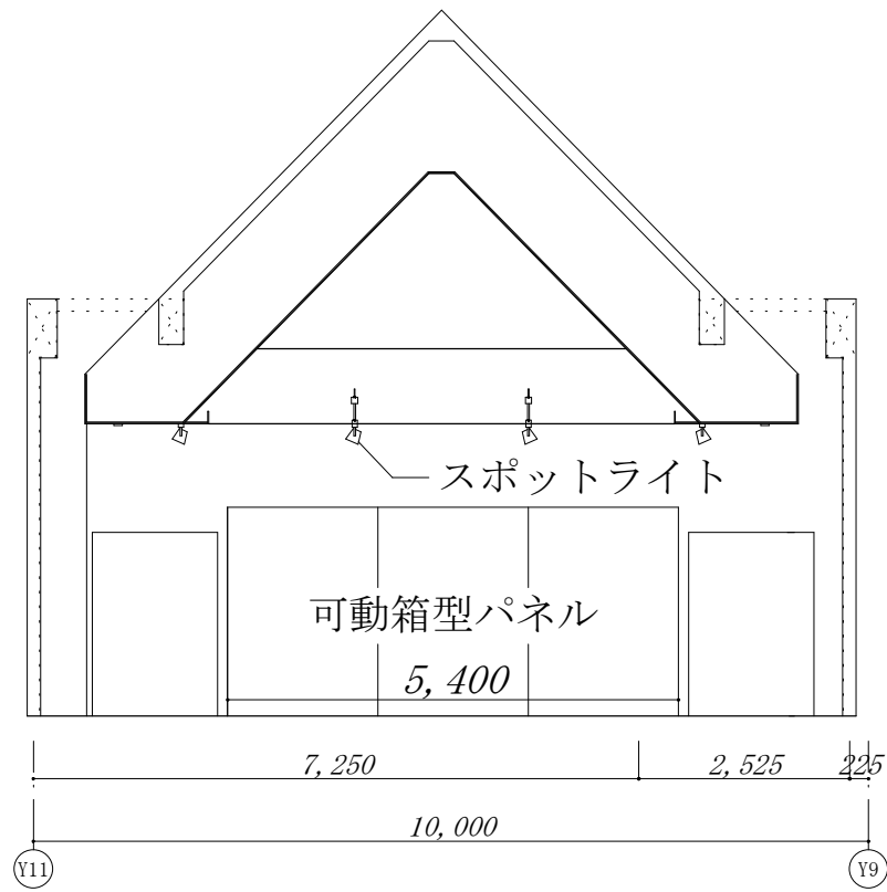
断面図
