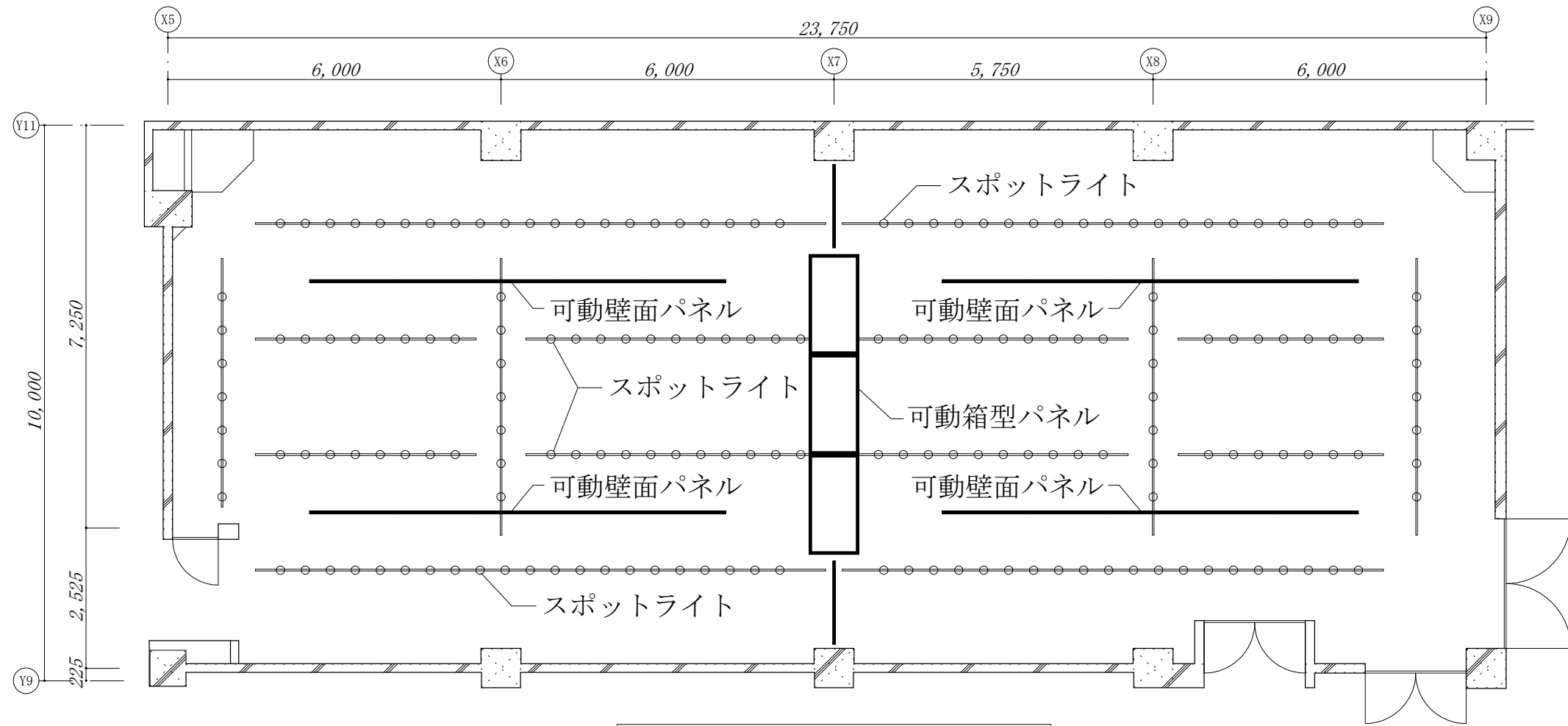
平面図
