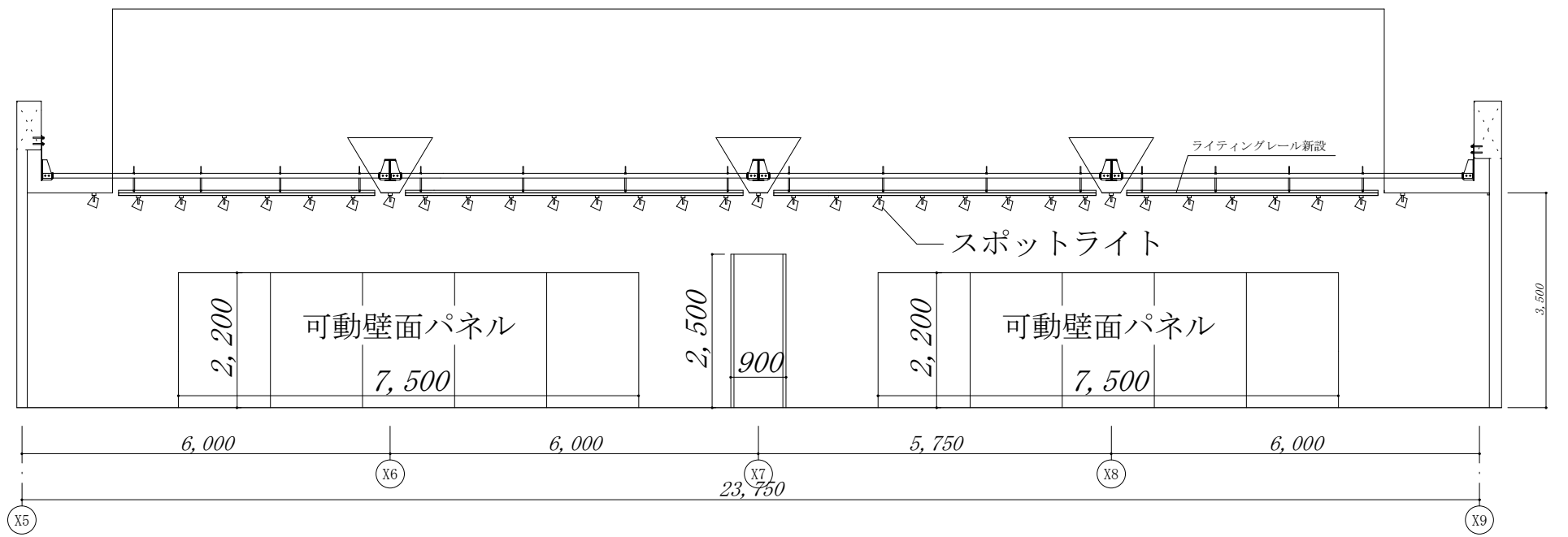
断面図
