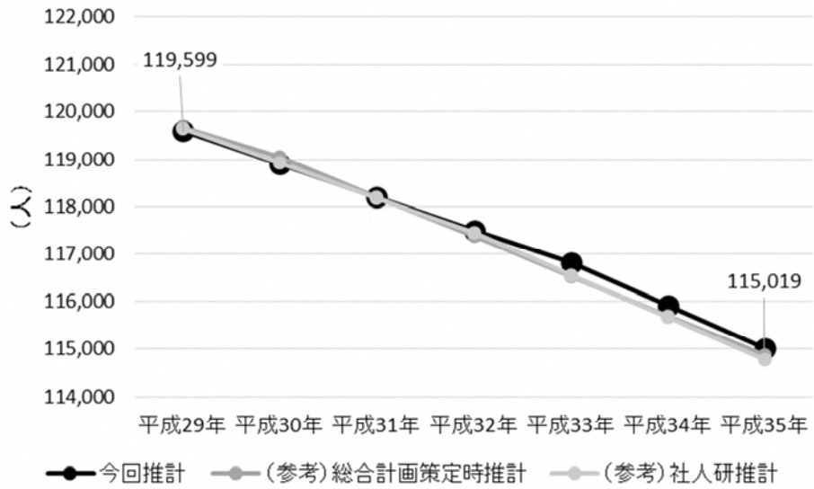
図表3 江別市将来人口推計結果（総合計画策定時推計及び社人研推計との比較）
