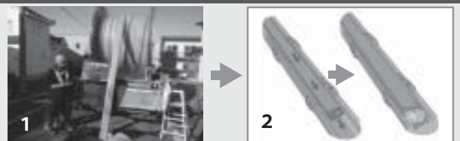
図2 新しい下水道管ができるまで <形成工法>
